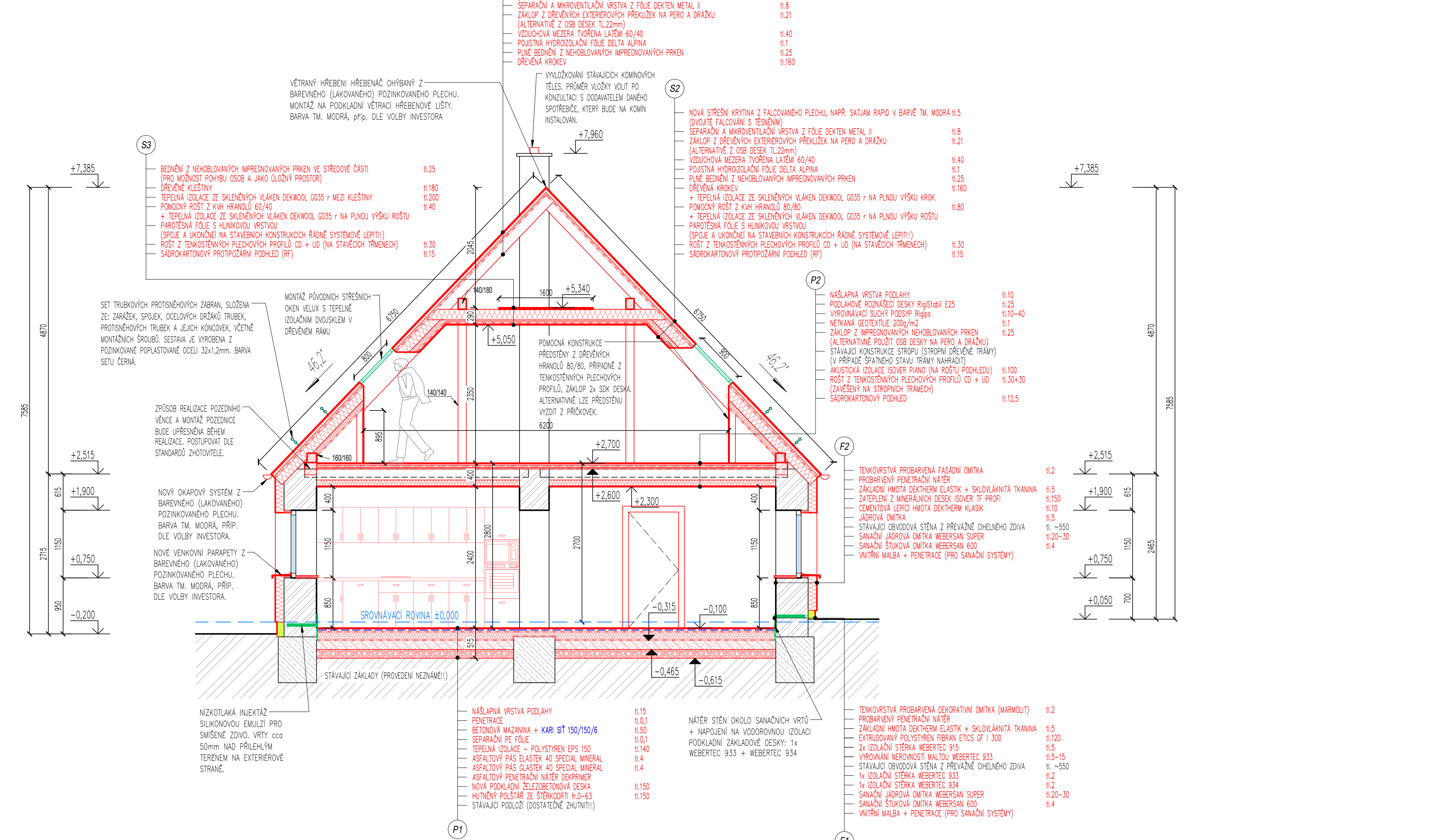
ŘEZ C-C - NOVÝ STAV
